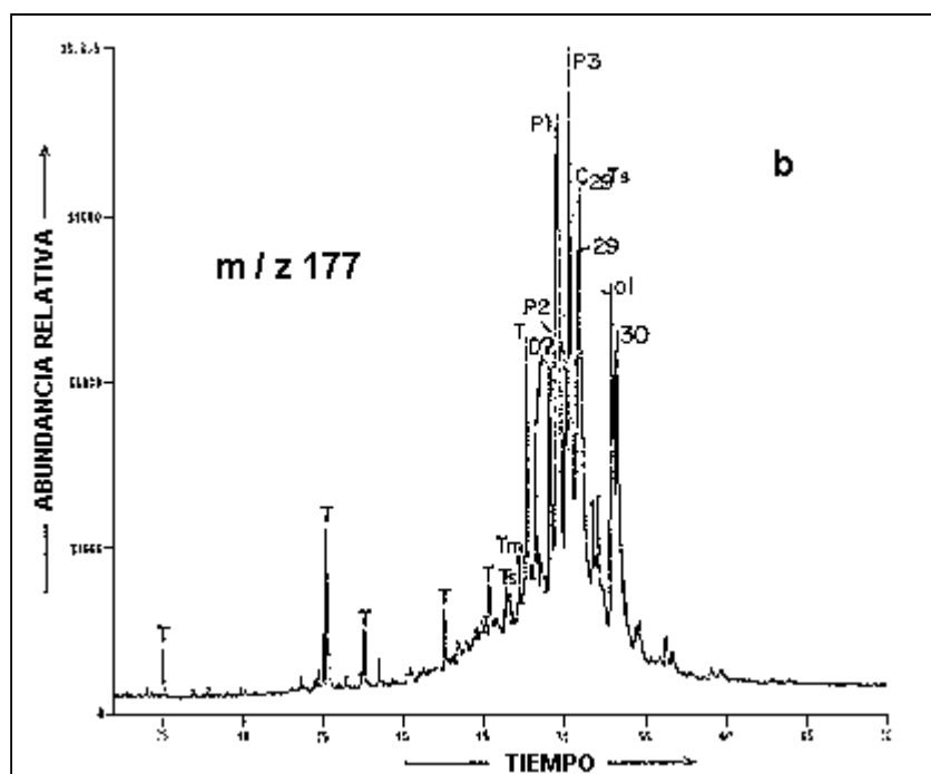
Distribución de biomarcadores terpanos m/z 191 (a) y m/z 177 (b) del Mene Cosme (Tomado de: Del Olio, 1993)
