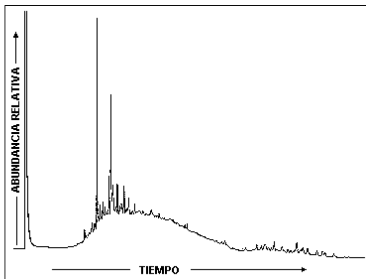
Cromatograma de la fracción saturada del Mene de Cosme (Tomado de: Del Olio, 1993)
