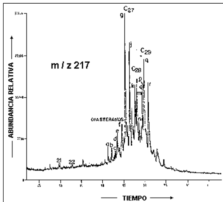
Distribución de biomarcadores esteranos m/z 217 Mene Cosme (Tomado de: Del Olio, 1993)
